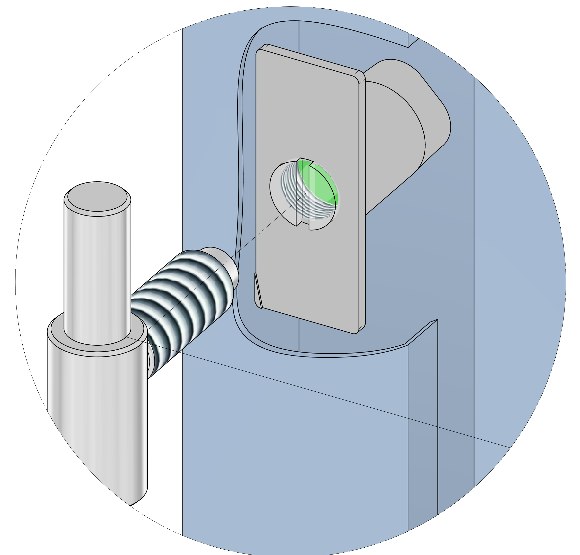
SZCZEGÓŁ "A"
